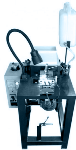
CODF90-2 ЭГЛЕТОЧНАЯ МАШИНА
